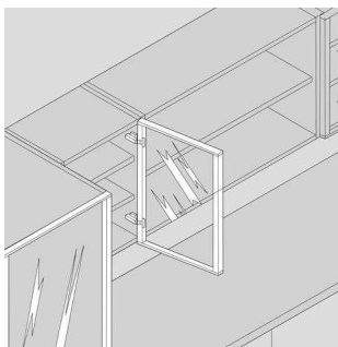
A410 لولای آرامبند استار پلاس تیتانیومی پروفیل آلومینیومی ۱۱۰ درجه روکار کلیپسی با پایه خطی 3D
