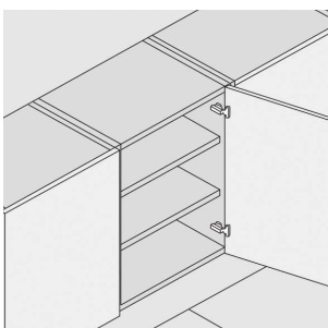
A124 لولای آرامبند پریمیوم تیتانیومی ۱۰۵ درجه روکار کلیپسی با پایه صلیبی 3D
