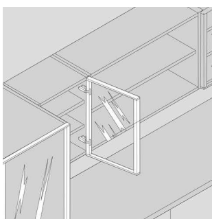
A115 لولای آرامبند پریمیوم پلاس پروفیل آلومینیومی ۹۵ درجه روکار کلیپسی با کاور مشکی و پایه خطی 3D
