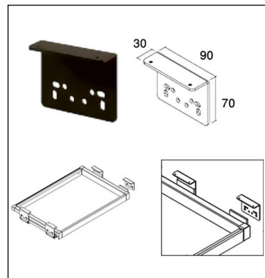
J483 بست ال زیر سقف جهت نصب رانر ریل
