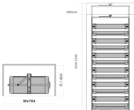
J949 | استند جا کفشی کمدی گردان طوسی فرنچ استایل عرض ۸۰۰mm
