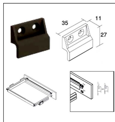
J484 بست اتصال اکسسوری ریلی طرح ویوو به درب چوبی
