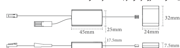
N807 سنسور چشمی درب کابینت و کمد روکار دو درب حداکثر ۴۸ وات
