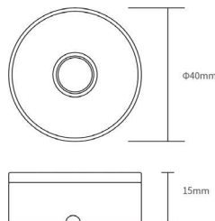
N677 چراغ LED گرد نقطه ای سه تایی همراه با ترانس به قطر 40mm
