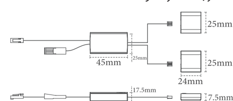
N808 سنسور چشمی درب کابینت و کمد روکار تک درب حداکثر ۴۸ وات
