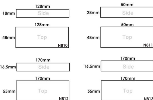
N813 ترانس یورو پلاگ ۶۰ وات ارتفاع ۱۶,۵mm، عمق ۵۵mm، عرض ۱۷۰mm Output voltage: DC12V Max. 5A
