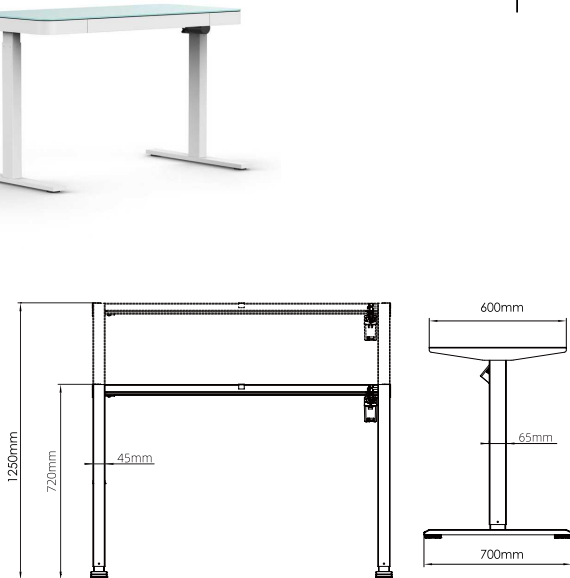
استند لیفت آپ دو پایه چند منظوره هوم آفیس | T102
